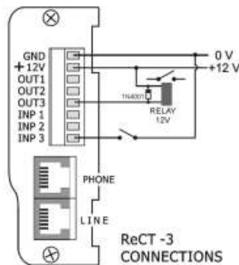
Σχήμα 1: Συνδέσεις του ReCT-3S
