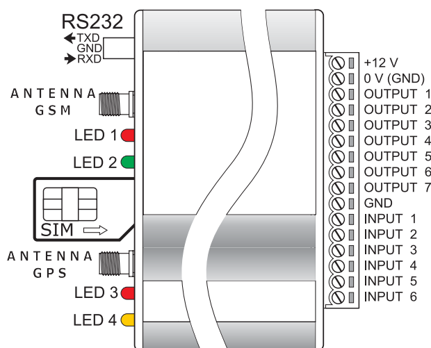
Σχήμα 1: Συνδέσεις του GMC 67
