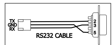
Σχήμα 2: Καλώδιο RS232
