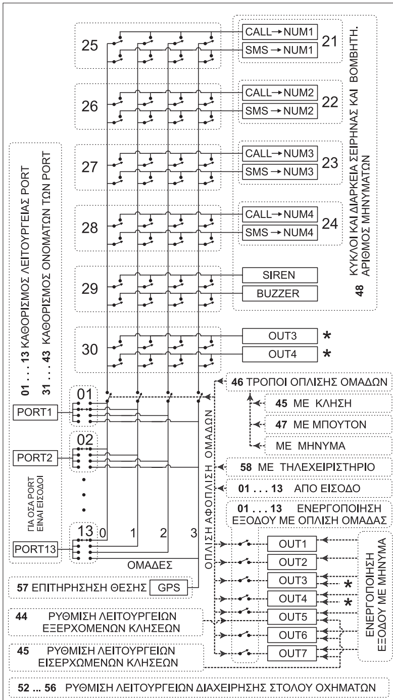
Σχήμα 3: Οι λειτουργίες του GMC και οι παράμετροι που τις ρυθμίζουν.
